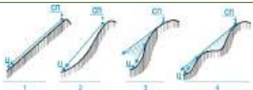
Іл. 30.10. Наявність взаємної видимості точок на одному схилі залежно від форми схилу
