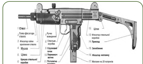
Іл. 19.17. Основні частини пістолета-кулемета UZI.
