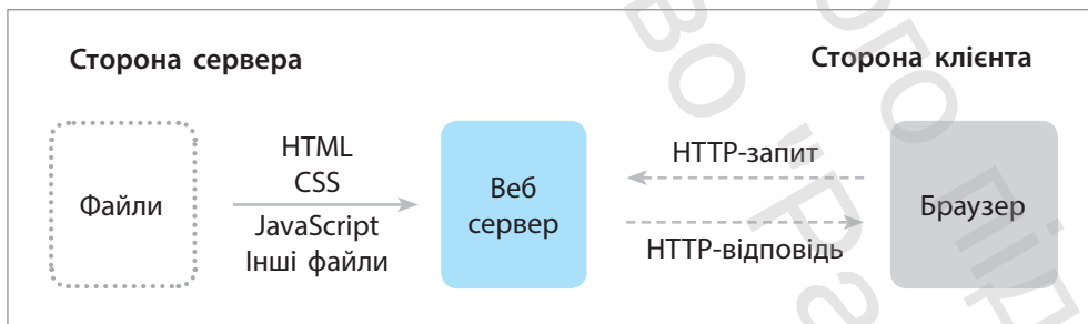
Рис. 11.88. Взаємодія «клієнт — сервер» на прикладі статичного сайта
