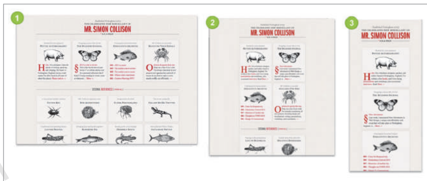
Рис. 11.58. Приклад адаптивної верстки на основі медіа-запитів
