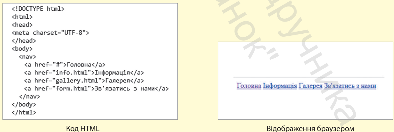
Рис. 11.37. Приклад запису навігаційного контейнера та його відображення браузером
