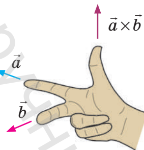
Рис. 10.6. Правило правої руки
