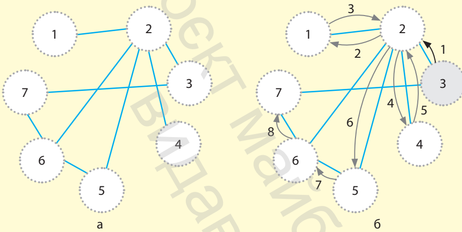
Рис. 8.16. Неорієнтований незважений граф (а), неорієнтований незважений граф, стрілкою позначено напрям руху, цифрою — номер кроку (б)
