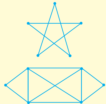
Приклади ейлерового графу
