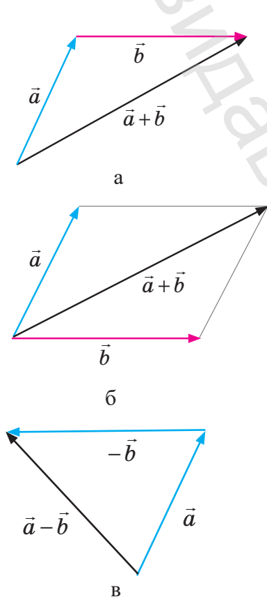
Рис. 10.4. Додавання і віднімання векторів
