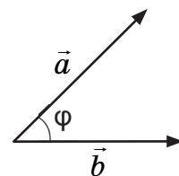
Рис. 10.8. Кут між векторами
