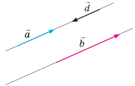
Рис. 10.3. Колінеарні вектори
