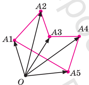
Рис. 10.11. П'ятикутник A_1A_2A_3A_4A_5
