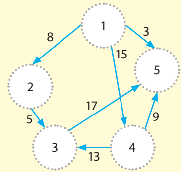
Рис. 8.14. Орієнтований зважений граф
