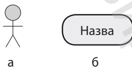
Рис. 12.9. Вигляд ектора (а) та прецедента (б)
