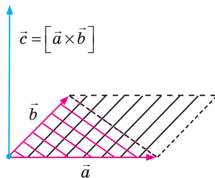
Рис. 10.5. Графічне зображення векторного добутку
