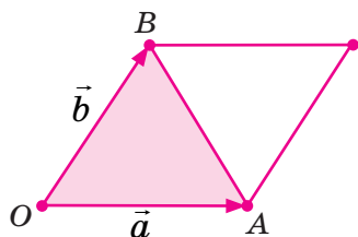
Рис. 10.12. Площа паралелограма, побудованого на двох векторах
