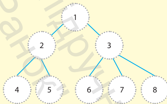
Рис. 8.7. Дерево (як вид графу)
