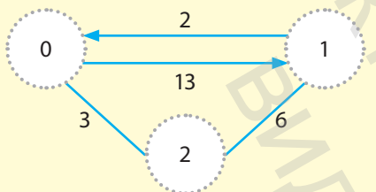
Рис. 8.22. Змішаний зважений граф
