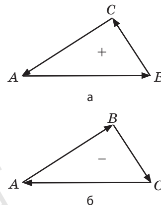
Рис. 10.9. Варіанти обходу вершин трикутника
