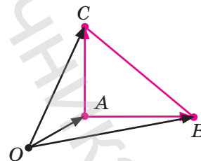
Рис. 10.10. Приклад обчислення орієнтованої площі трикутника
