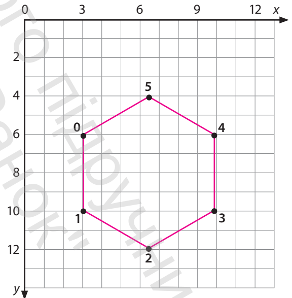
Рис. 10.14. Результат виконання програми — многокутник за заданими координатами
