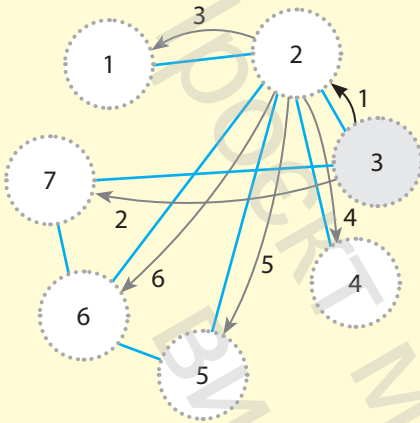
Рис. 8.16, в. Неорієнтований незважений граф, стрілкою позначено напрям руху, цифрою — номер кроку
