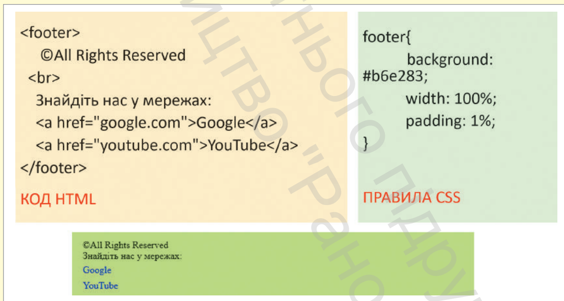
Рис. 11.48. Нижній колонтитул вебсторінки
