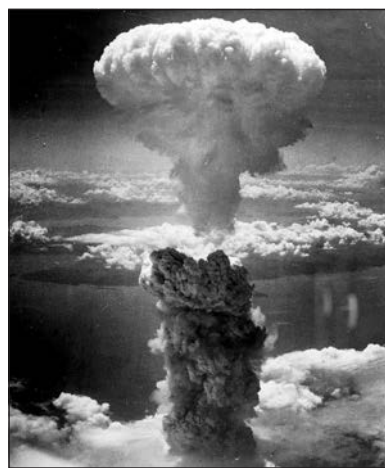
Вибух атомної бомби, скинутої на Нагасакі 9 серпня 1945 р.
